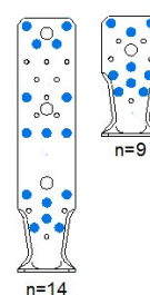
Clouage partiel
