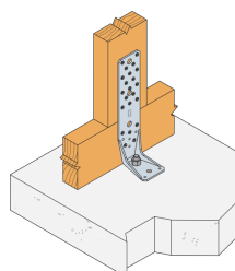
Plan de clouage sur poteau
